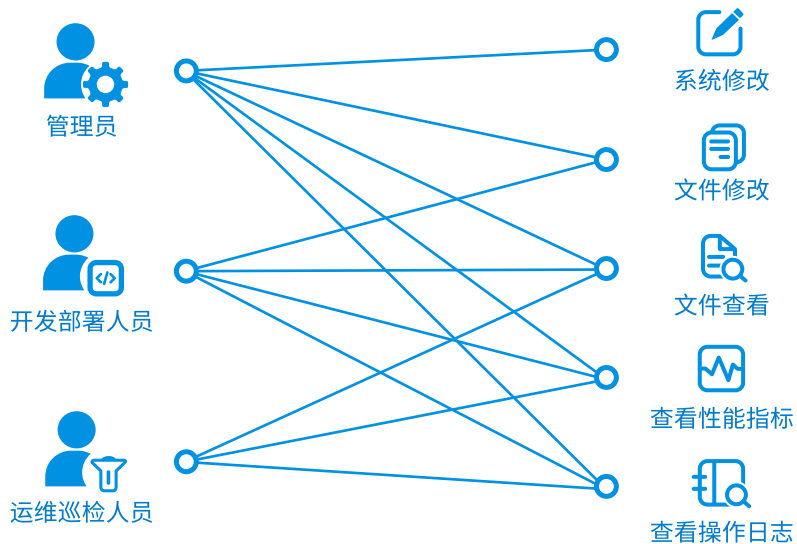
图表七 操作系统安全
